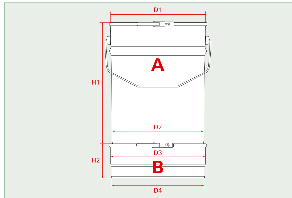
Wymiary standardowe Komponent A
